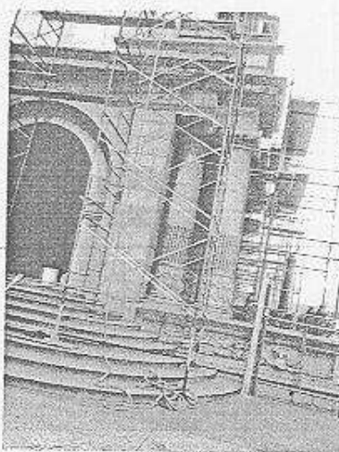
Inicio de la Instalación del andamio nuevo en la Parte Sur Este del Torreón Central y personal trabajando en forma segura
