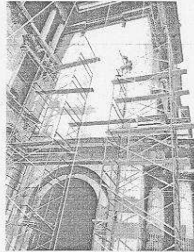
Las cuerdas que sirven para asegurar el andamio y también una cuerda salvavidas en caso de emergencia
